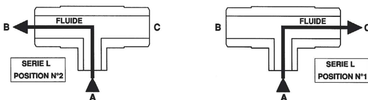
Vanne à boisseau sphérique 3 voies en L VBS 3VL
