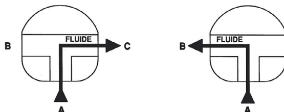
Robinet à boisseau cylindrique RBC 3VL
