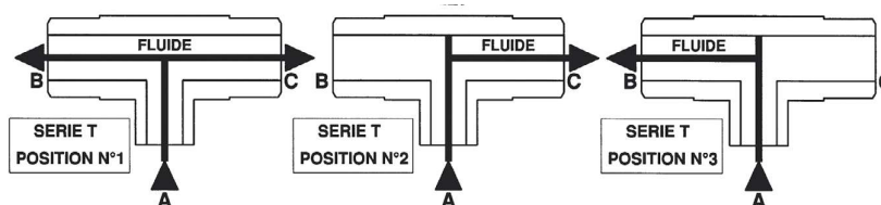
Vanne à boisseau sphérique 3 voies en T VBS 3VT
